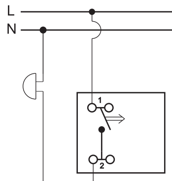
Schemat podłączenia wyłącznika zwiernego.
